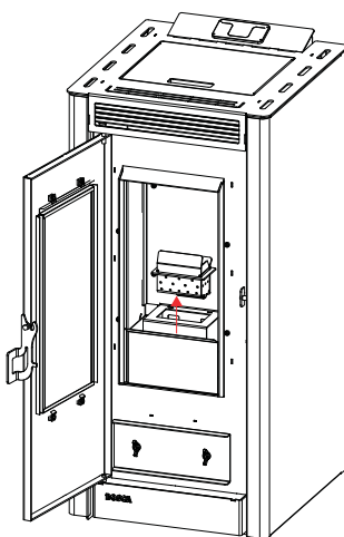
EXTRACCION QUEMADOR PARA LIMPIEZA
