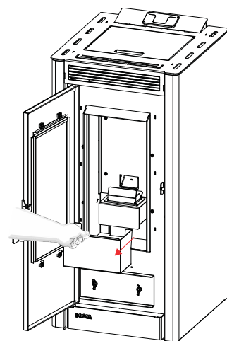
EXTRACCION CENIZERO PARA LIMPIEZA
